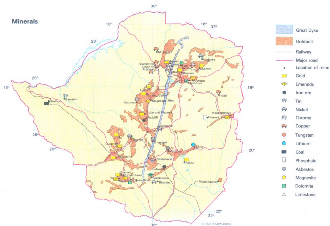
Карта полезных ископаемых Зимбабве.
