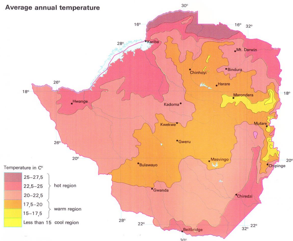
Карта среднегодовых температур
